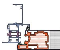
Dormant standard aile de 15 (pose en applique avec tapées)
