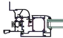
Dormant à recouvrement (sur dormant existant)
